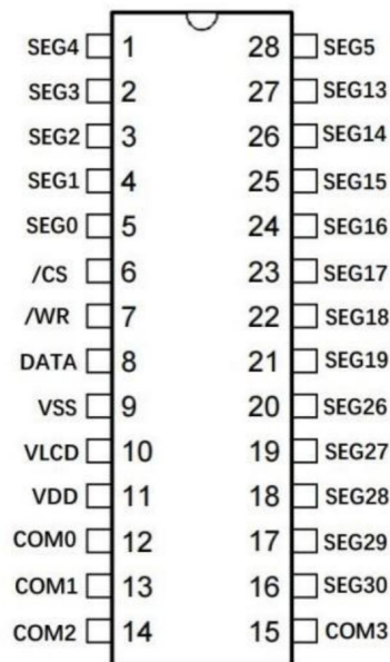
SSOP-28
